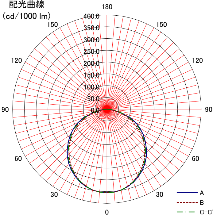
配光曲線
